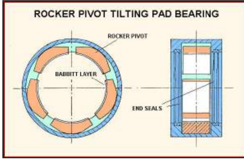
الكرسى ذو الوسائد المائلة TILTING PAD BEARING
